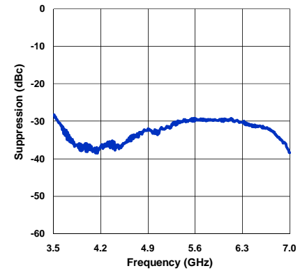
Sideband Suppression
