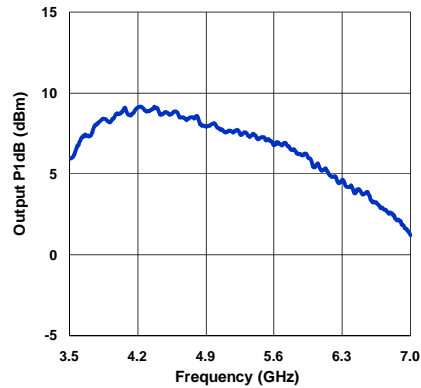
Output P1dB
