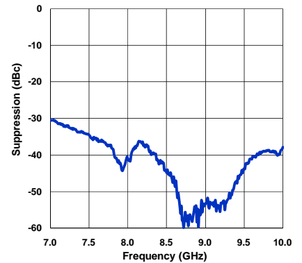
Sideband Suppression
