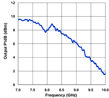
Output P1dB
