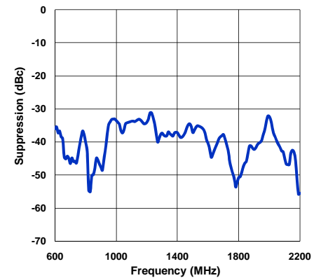
Sideband Suppression
