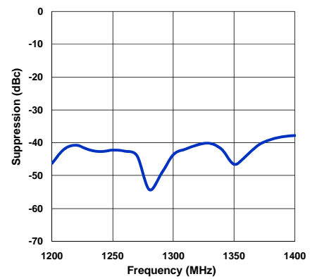
Sideband Suppression
