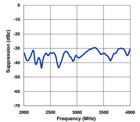
Sideband Suppression
