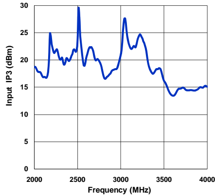
Input IP3
